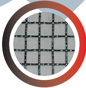
38 mm göz ( atlamalı ) ( Tel \varnothing 8 mm ) eleme alanı : % 57 - 68 m
