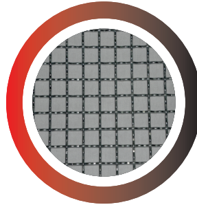
45 mm göz ( Tel \varnothing 8 mm ) eleme alanı : % 58 - 70 m tek atkılı
