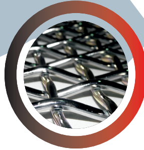
30 mm göz ( Tel \varnothing 8 mm ) eleme alanı : % 59 - 68 m
