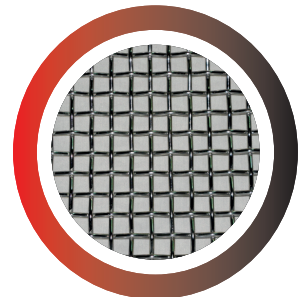
19 mm göz ( Tel \varnothing 5 mm ) eleme alanı : % 55 - 61 m
