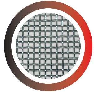
15 mm göz ( Tel \varnothing 5 mm ) eleme alanı : % 55 - 62 m
